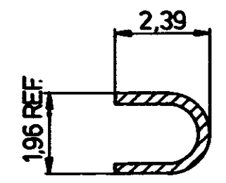
SCHNITT C-D
