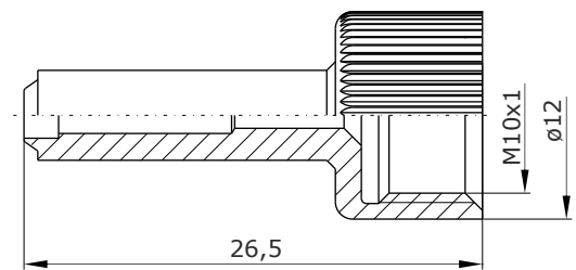
Hauptabmessungen Ausbauhülse
