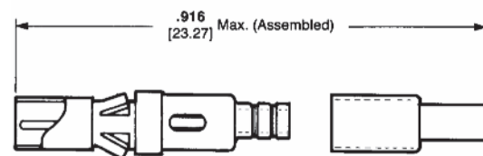
Cable Socket
