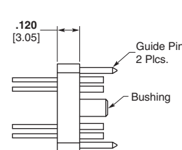
Receptacle
