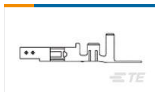
TE Part #1586315-1 VAL-U-LOK SKT BR SN 24-18 LP
