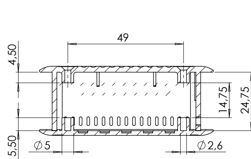
SEZIONE A-A
