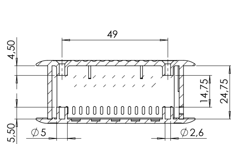
SEZIONE A-A
