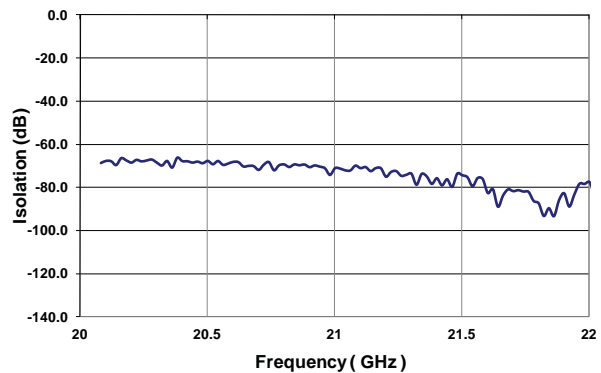
Isolation (20-22 GHz)
