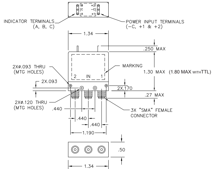
Optional Narrow Width Body
