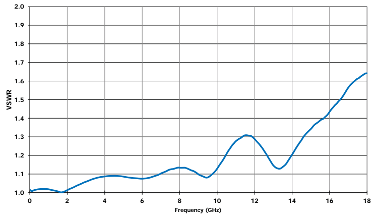
VSWR (DC - 18GHz)
