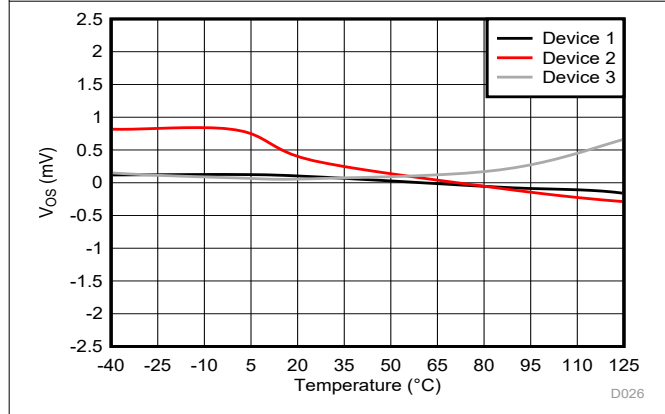
图 6-9. Input Offset Voltage vs Temperature
