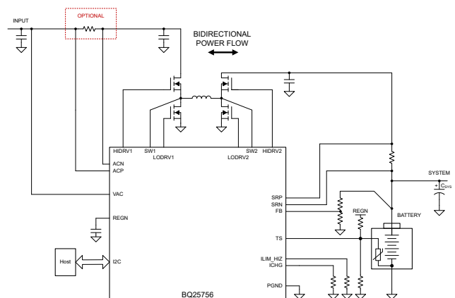
简化原理图
