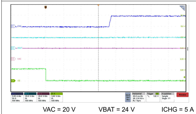
图 9-7. Charge Enable via \overline{\text{CE}} Pin with 5-A ICHG
