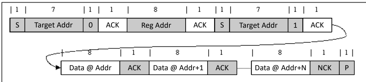
图 8-15. Multi-Read
