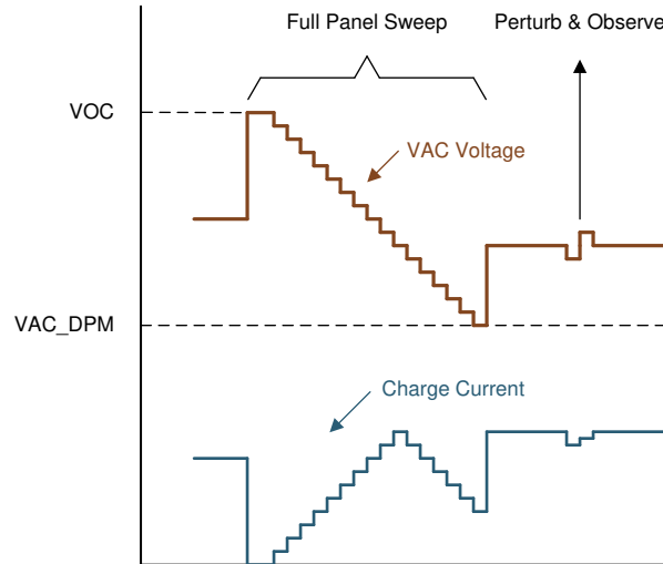
图 8-6. Maximum Power Point Tracking
