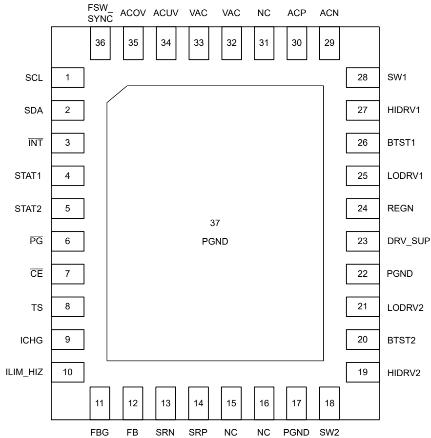
图 6-1. BQ25756, RRV Package 36-pin VQFN Top View
