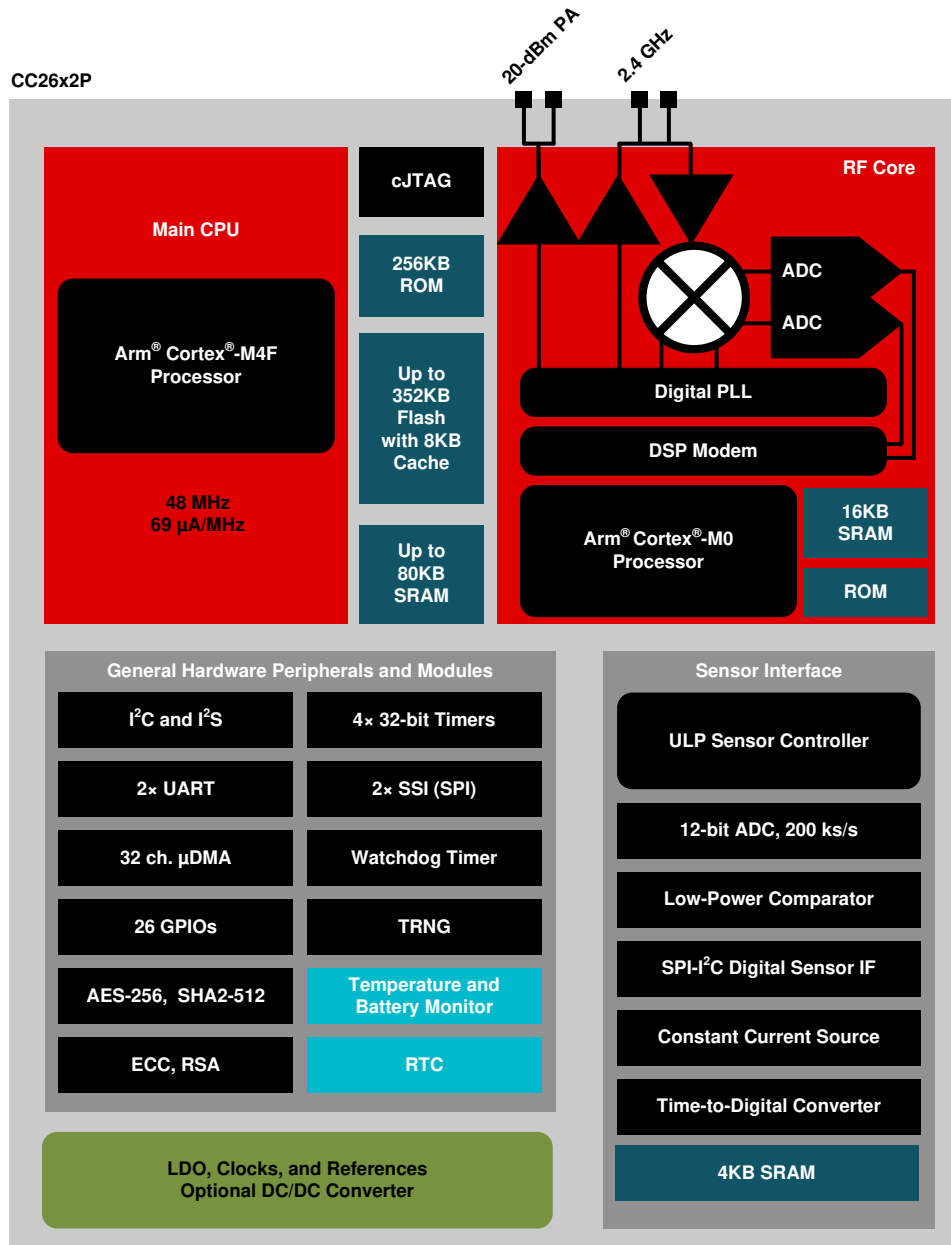
图 4-1. CC2652P Block Diagram
