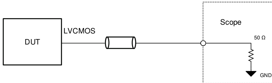
图 8-2. LVCMOS Output Test Configuration
