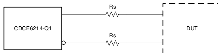
图 8-14. LP-HCSL Output
