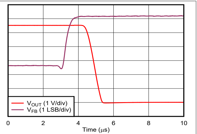
图 6-52. 比较器响应时间：高电平到低电平转换
