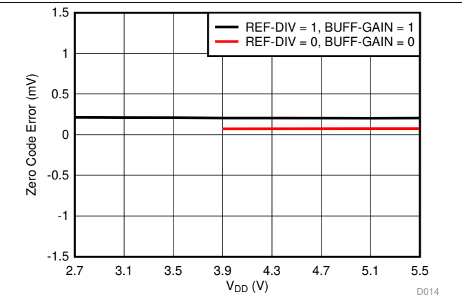
图 16. Zero Code Error vs Supply Voltage
