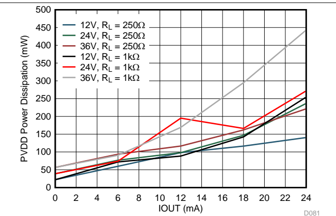
图 83. IOUT Power Dissipation vs Load
