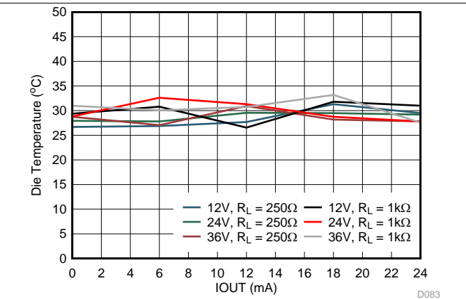
图 85. IOUT Die Temperature vs Load
