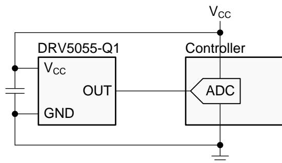
典型原理图
