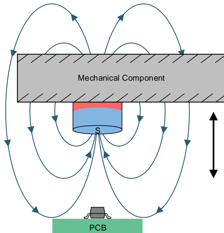
图 20. Physical Setup
