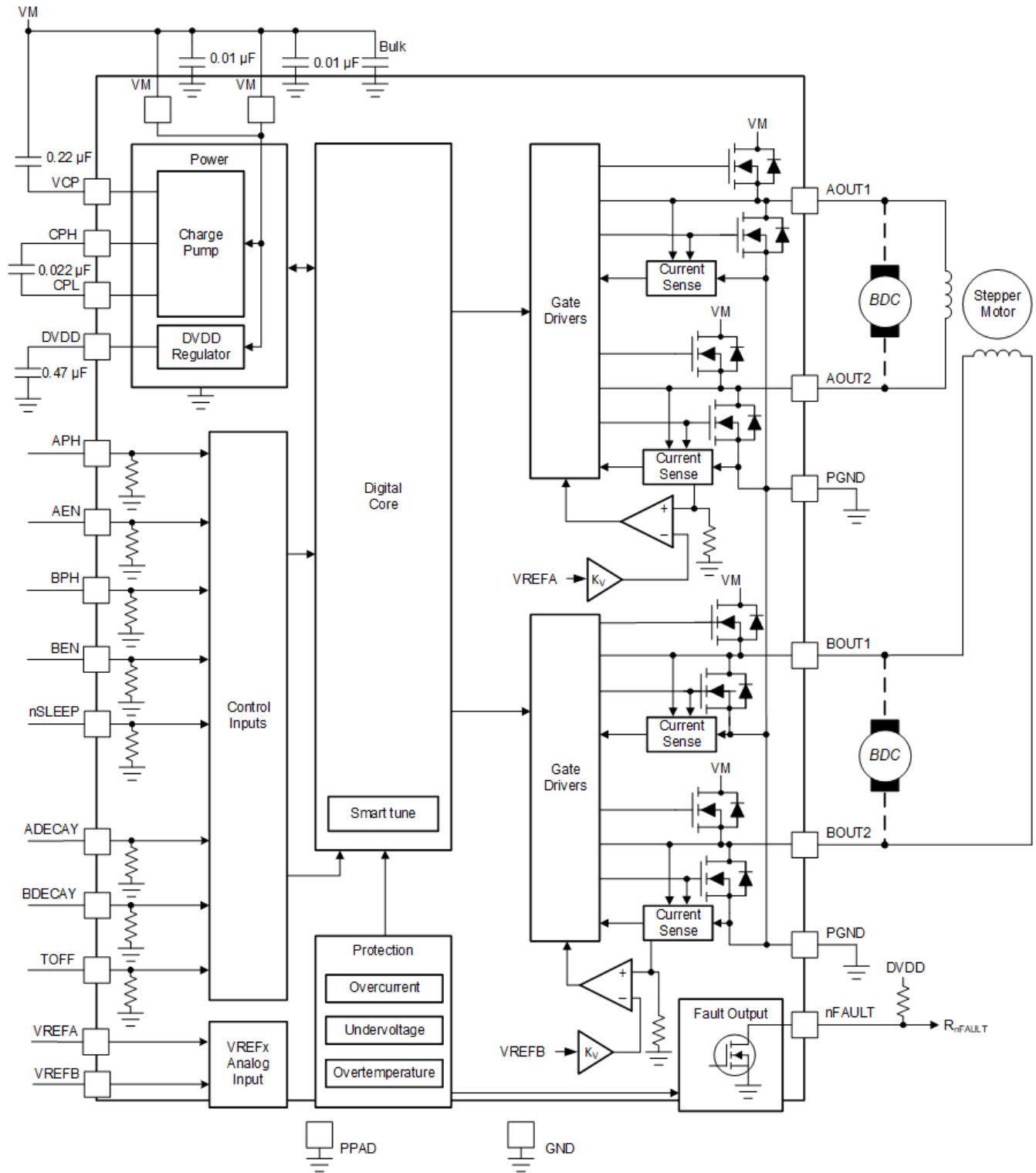
图 7-1. DRV8424E、DRV8425E 方框图
