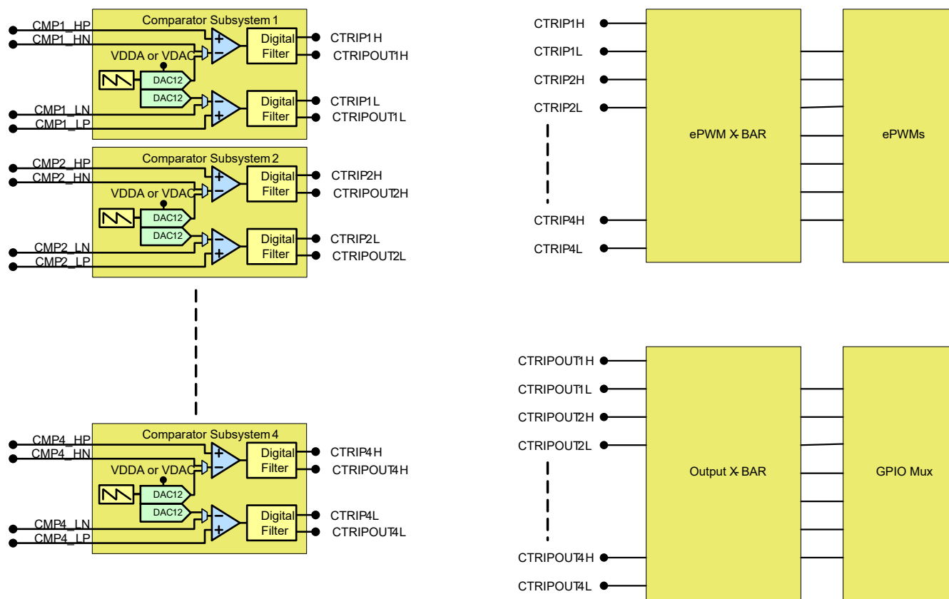
图 6-41. CMPSS Connectivity
