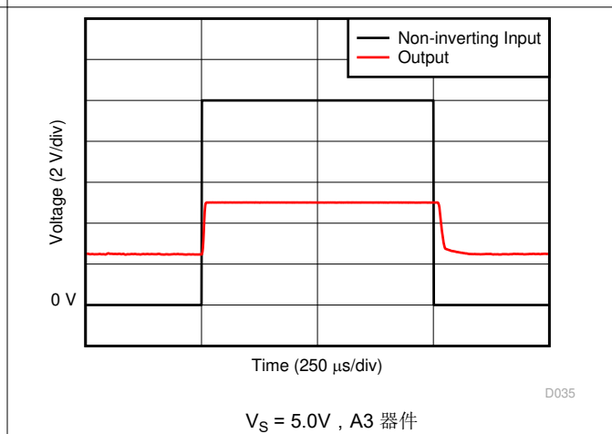
图 6-16. 同相差分输入过载
