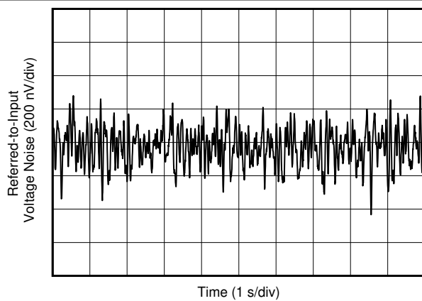
图 6-25. Input Referred Noise
