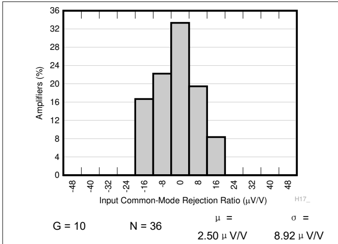
图 7-7. CMRR 的典型分布
