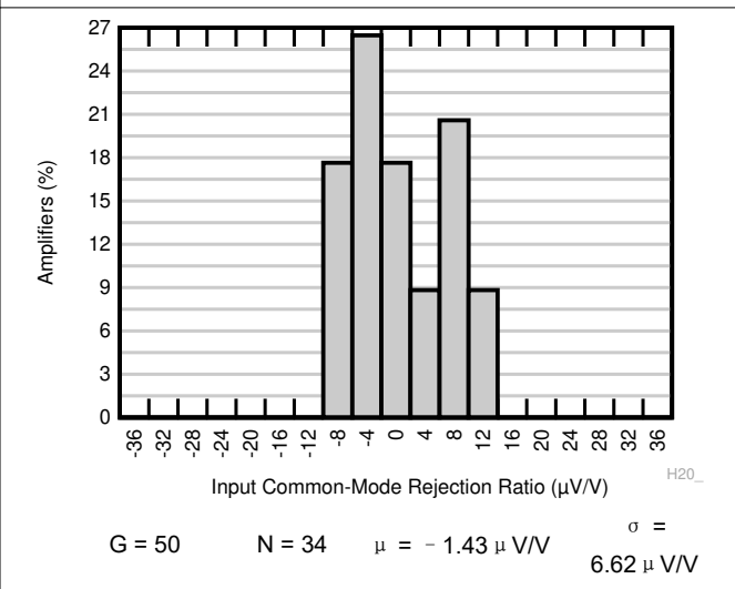
图 7-10. CMRR 的典型分布
