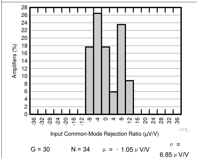
图 7-9. CMRR 的典型分布
