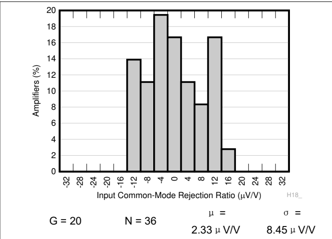
图 7-8. CMRR 的典型分布
