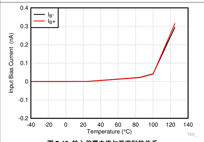
图 7-12. 输入偏置电流与温度间的关系
