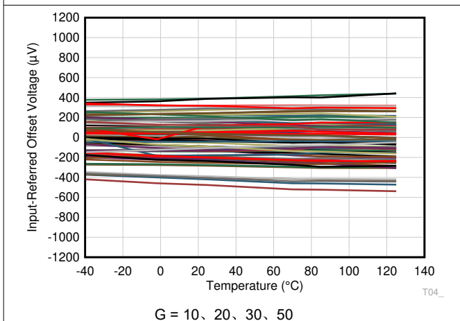
图 7-11. 输入参考失调电压与温度间的关系
