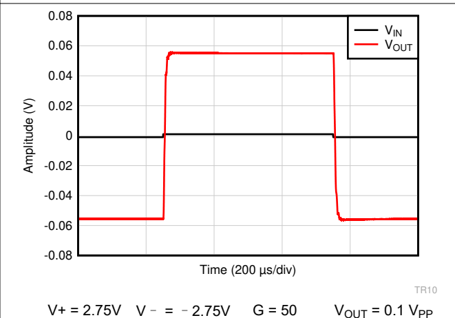
图 7-46. 小信号阶跃响应
