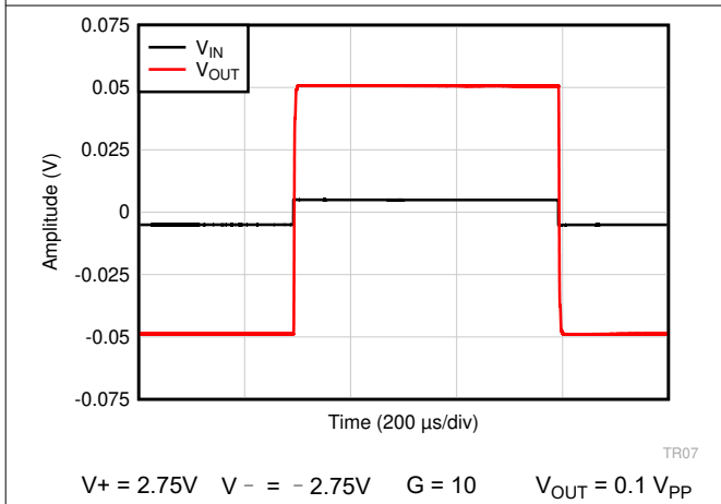
图 7-45. 小信号阶跃响应
