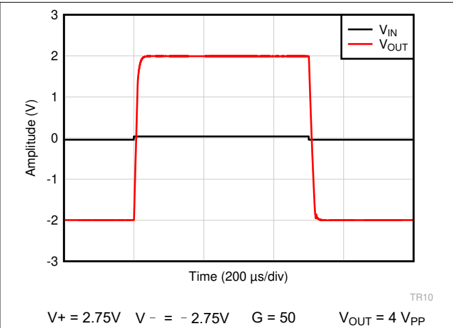
图 7-44. 大信号阶跃响应
