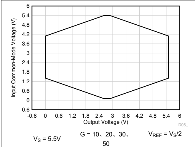
图 7-57. 输入共模电压与输出电压间的关系
