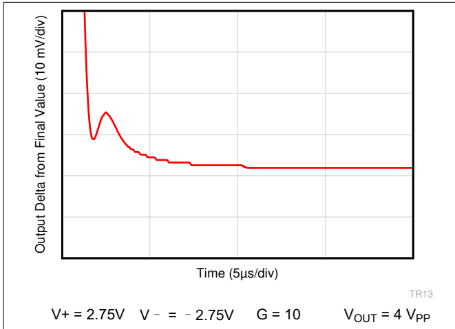
图 7-43. 大信号稳定时间 (上升沿)
