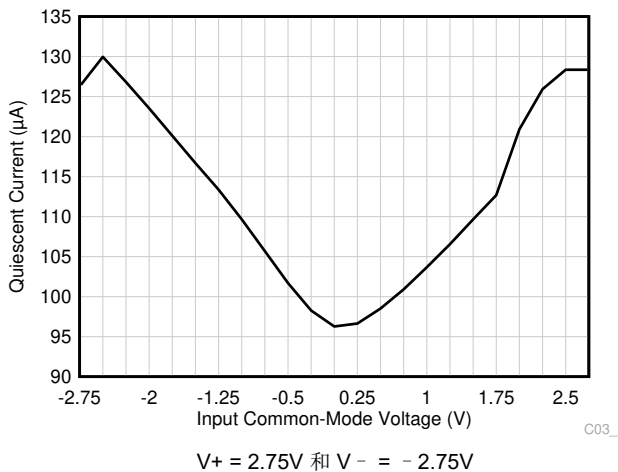
图 7-23. 静态电流与输入共模电压间的关系
