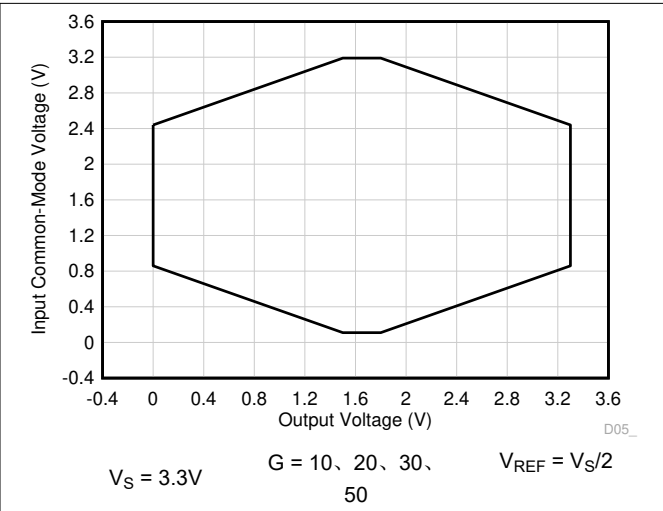
图 7-56. 输入共模电压与输出电压间的关系
