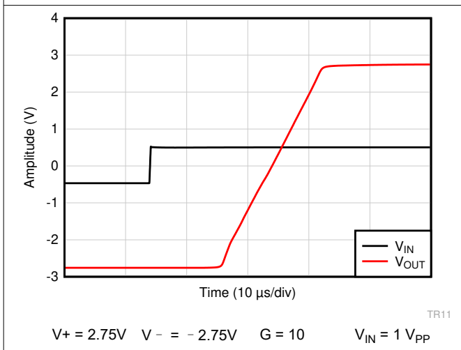
图 7-47. 过载恢复 (上升沿)
