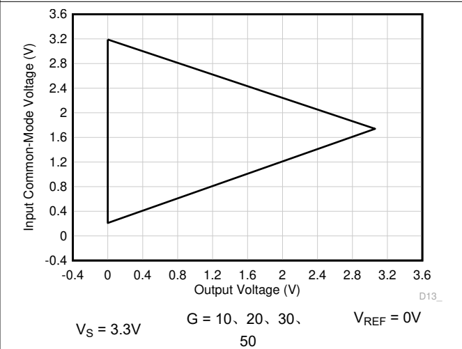
图 7-58. 输入共模电压与输出电压间的关系
