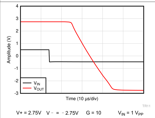
图 7-48. 过载恢复 (下降沿)
