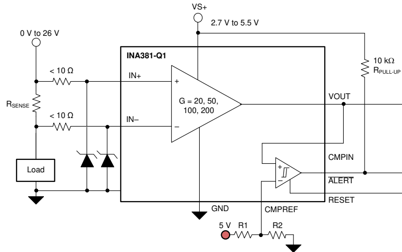
图 8-2. 瞬态保护
