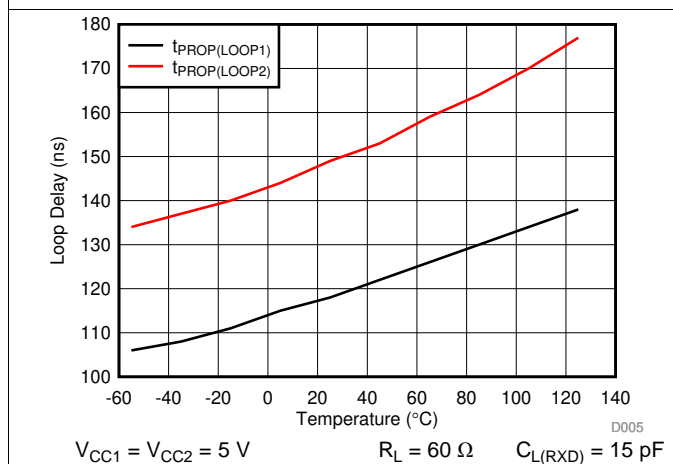
图 9. Loop Delay vs Ambient Temperature
