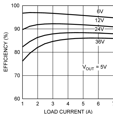
典型应用电路效率
