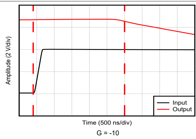
图 6-22. 过载恢复 (正轨)
