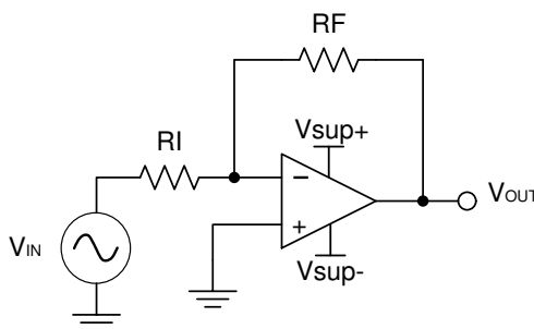
图 10-1. 应用原理图
