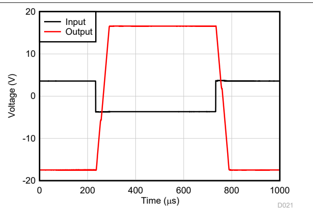
图 7-28. 过载恢复
