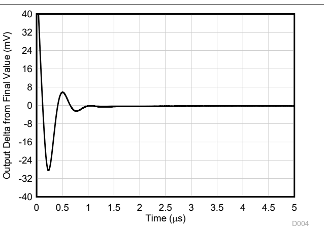
图 7-30. 小信号阶跃响应, G = -1
