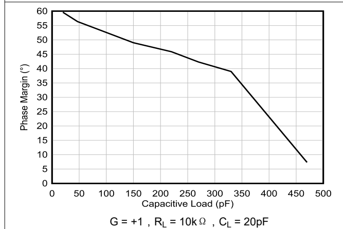
图 6-21. 相位裕度与容性负载间的关系
