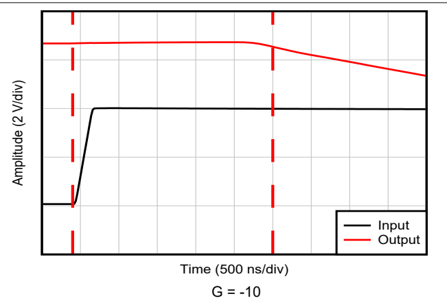
图 6-22. 过载恢复 (正轨)
