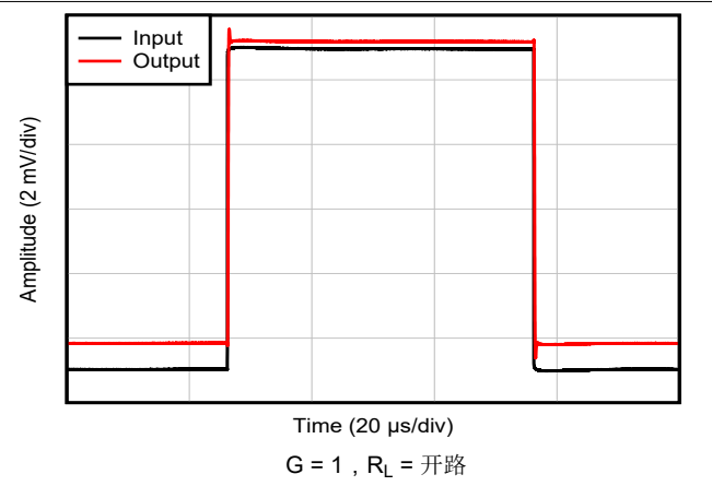
图 6-24. 小信号阶跃响应, G = 1
