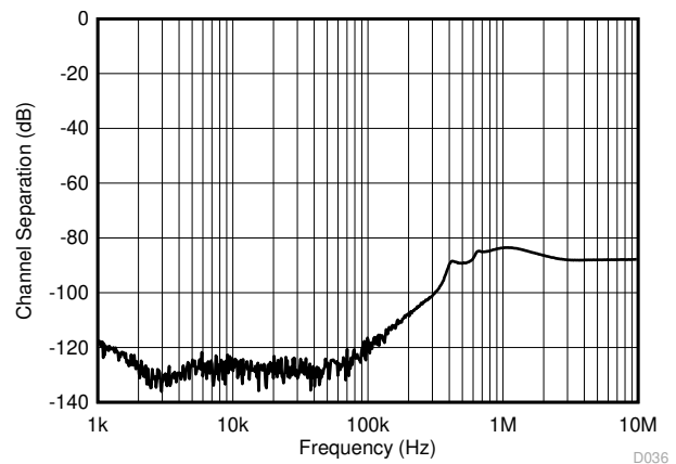
图 6-29. 通道分离
