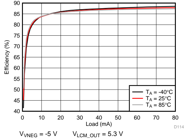
图 164. VNEG Efficiency
