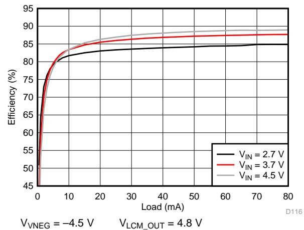
图 166. VNEG Efficiency
