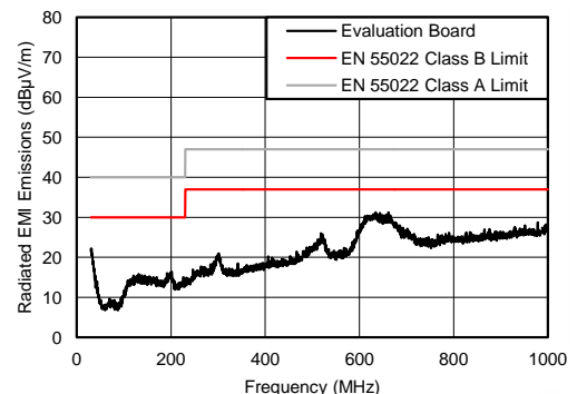
LM43602PWPEVM 辐射发射图 12 V_{IN} 至 3.3 V_{OUT} , F_S = 500kHz , I_{OUT} = 2A
