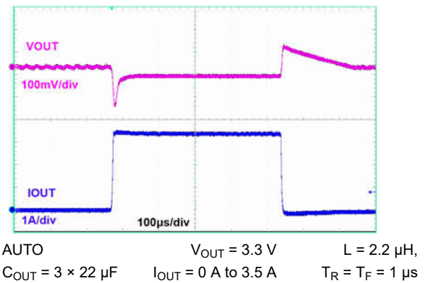
图 9-30. Load Transient
