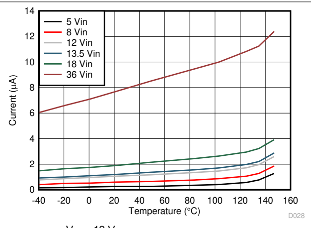
图 7-6. Shutdown Current
