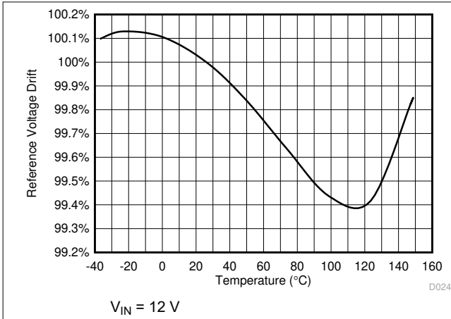
图 7-1. Reference Voltage Drift
