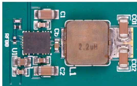
典型车用布局 (22mm \times 12.5mm)
