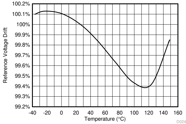
图 7-1. Reference Voltage Drift
