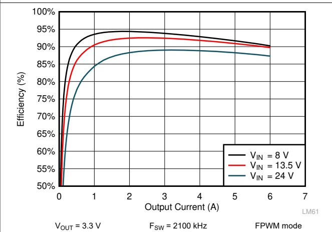
图 9-10. LM61460 Efficiency
