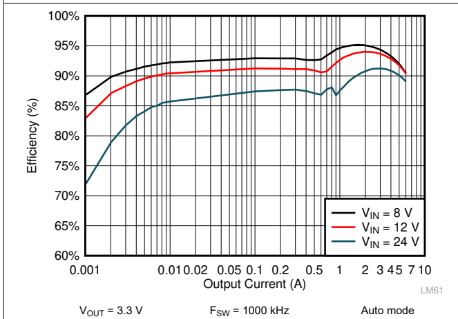
图 9-7. LM61460 Efficiency
