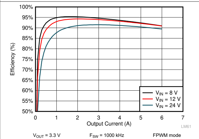
图 9-8. LM61460 Efficiency
