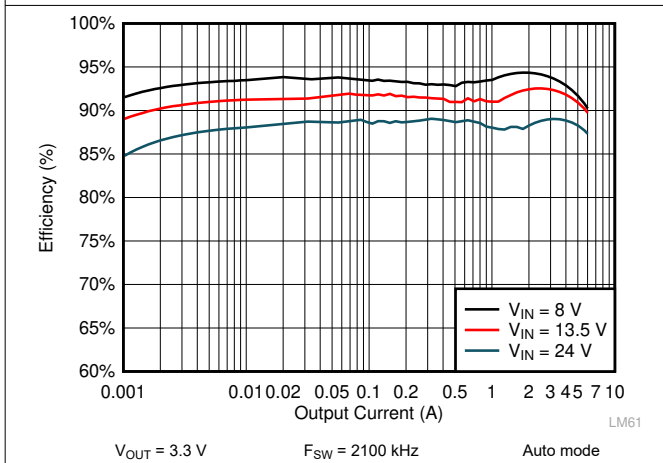
图 9-9. LM61460 Efficiency
