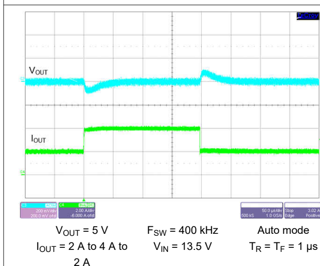
图 9-39. Load Transient
