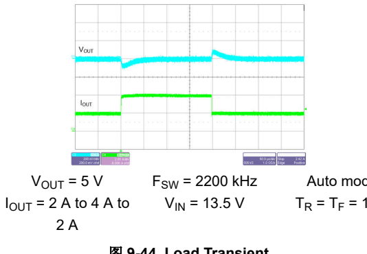
图 9-44. Load Transient
