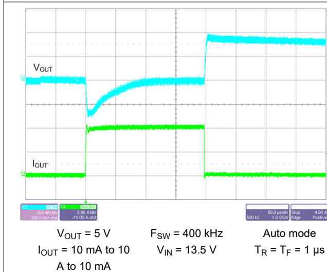
图 9-37. Load Transient
