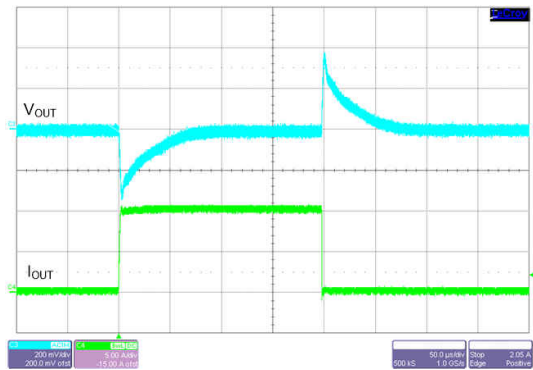
图 9-41. Load Transient
