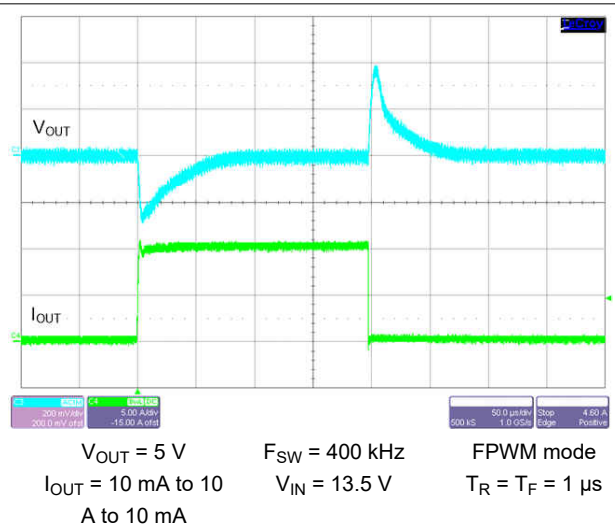
图 9-38. Load Transient
