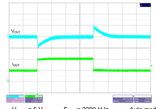
图 9-43. Load Transient
