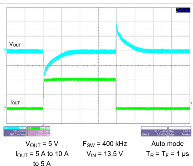
图 9-40. Load Transient
