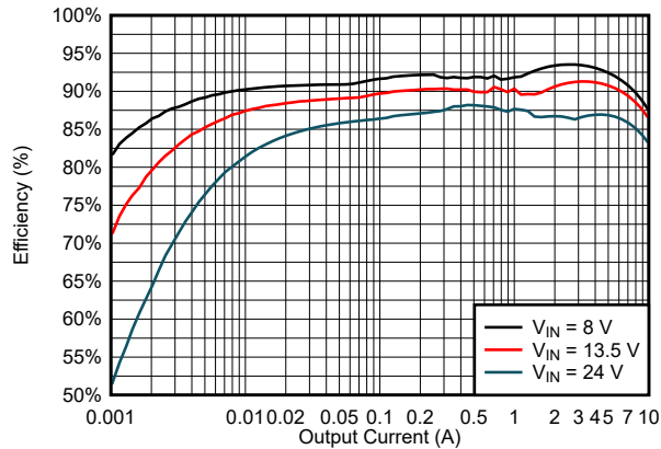
图 9-11. Efficiency
