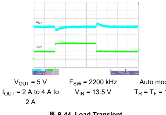
图 9-44. Load Transient
