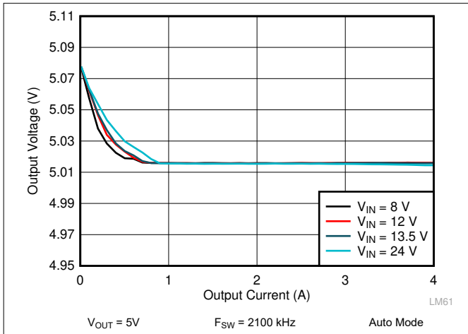
图 10-11. LM62440-Q1 Load and Line Regulation
