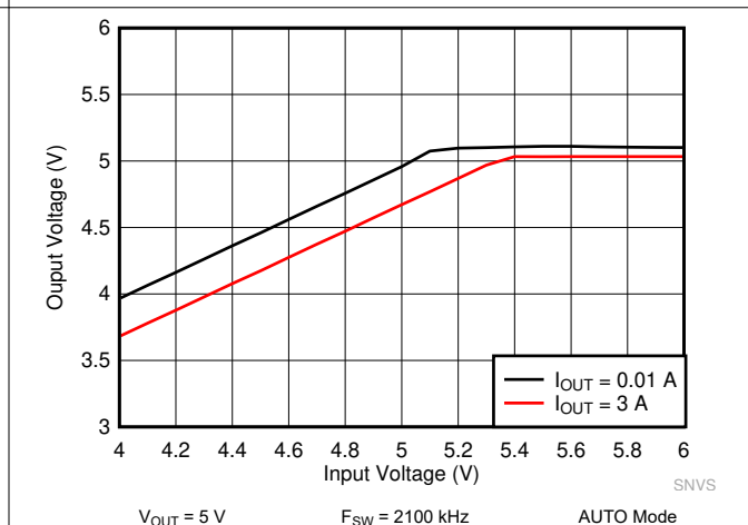
图 10-14. LM62440-Q1 Dropout Curve
