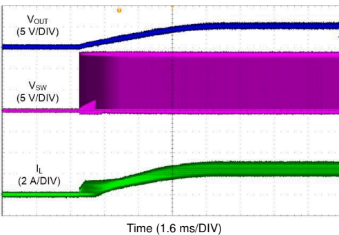
图 10-19. LM62440-Q1 Start-up with 3.25-A
