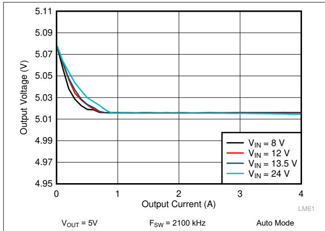
图 10-11. LM62440-Q1 Load and Line Regulation
