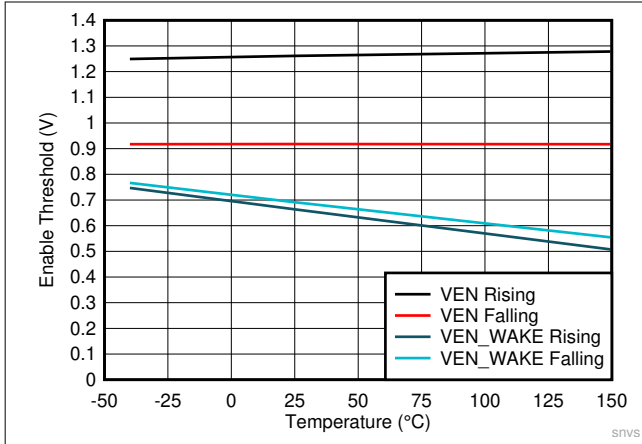
图 8-7. Enable Thresholds
