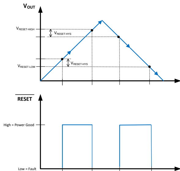
图 8-4. 静态 \overline{RESET} 操作
