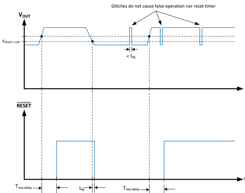
图 8-5. \overline{RESET} 时序行为
