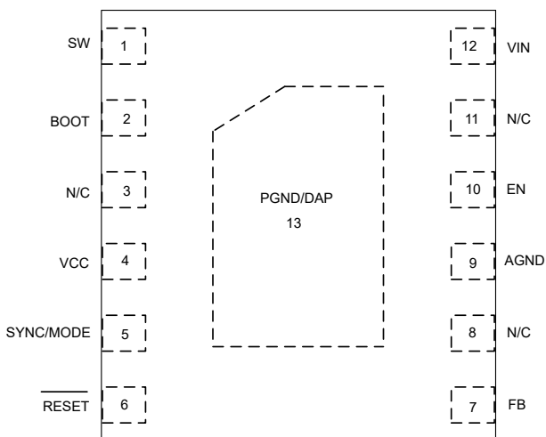
图 6-3. 采用 PowerPad 的 12 引脚 WSON DRR 封装 — LM636x5C (顶视图)
