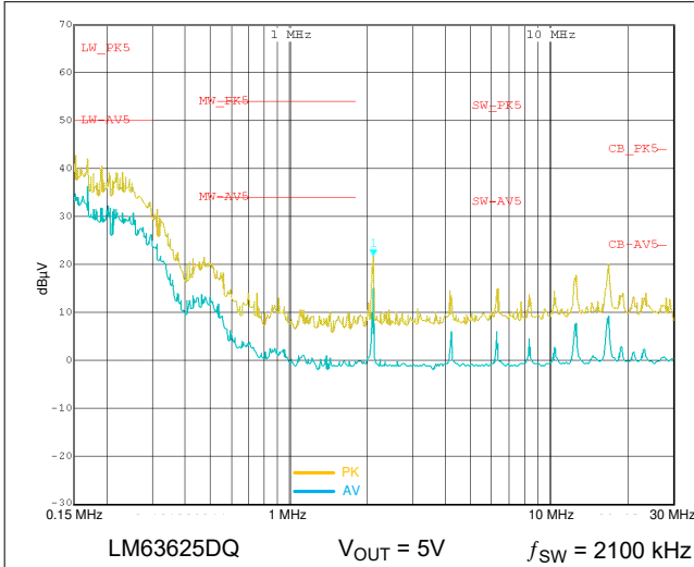
图 9-45. 典型传导 EMI 为 0.15MHz 至 30MHz
