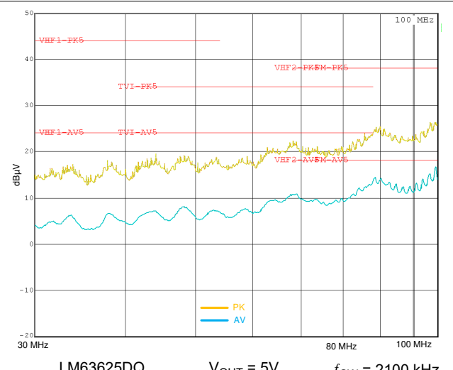
图 9-46. 典型传导 EMI 为 30MHz 至 108MHz
