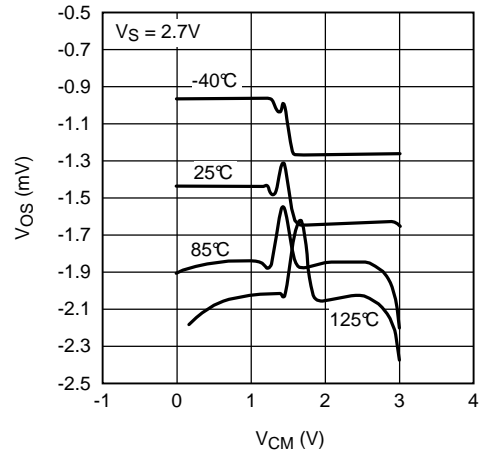
图 10. V_{OS} 与 V_{CM} 间的关系 (单位 3)
