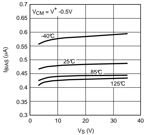
Figure 27. I_{BIAS} vs. V_S
