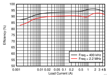
效率与负载电流 V_{OUT} = 5\text{V} , V_{IN} = 12\text{V} , 自动模式
