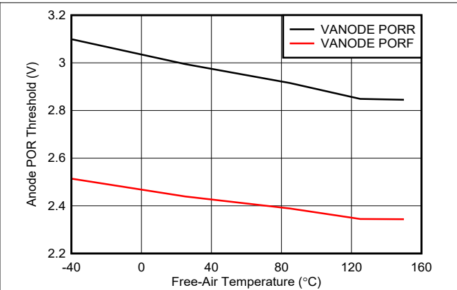
图 6-14. V_{ANODE} POR Threshold vs Temperature
