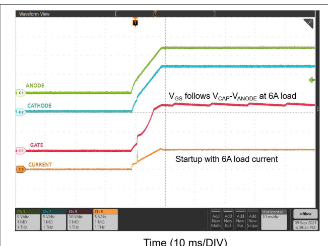
图 9-11. Startup With 6-A Load
