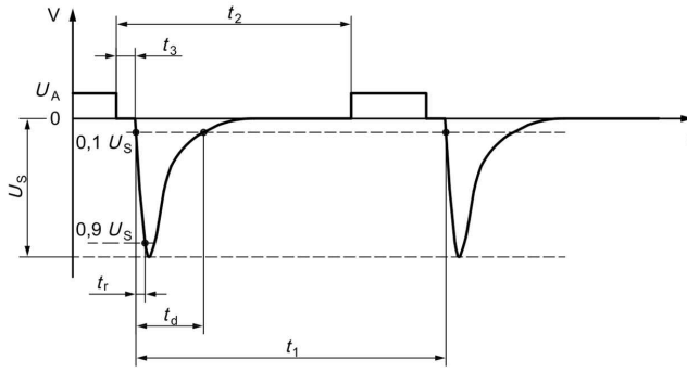
图 9-4. ISO 7637-2 Pulse 1
