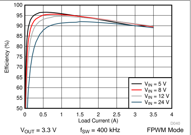
图 24. LM76003-Q1 Efficiency
