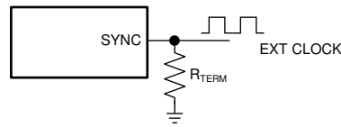
图 18. Frequency Synchronization
