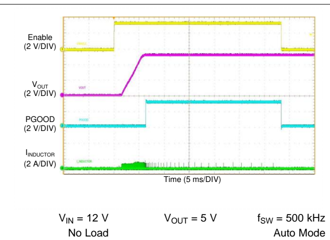
图 64. LM76003-Q1 Start-up Waveform
