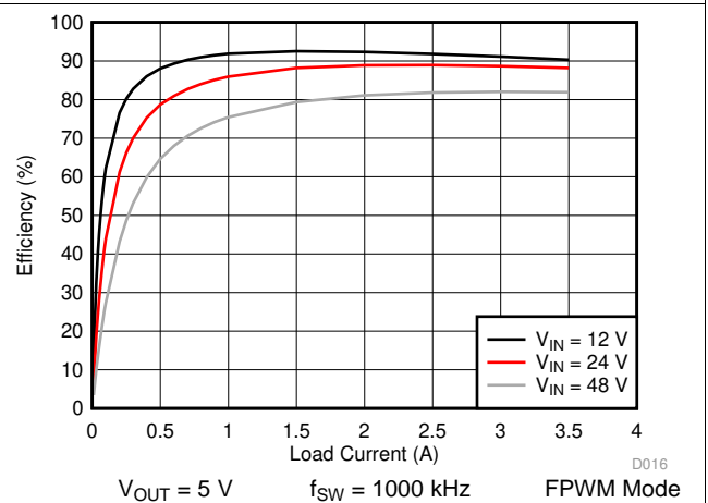
图 28. LM76003-Q1 Efficiency
