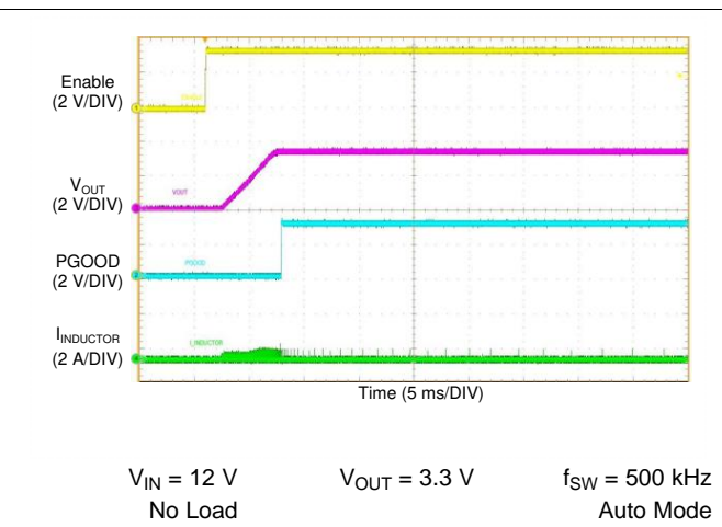
图 62. LM76003-Q1 Start-up Waveform
