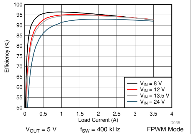
图 26. LM76003-Q1 Efficiency
