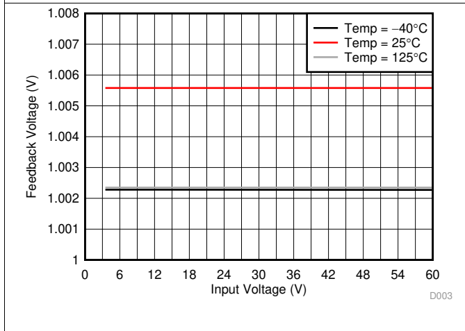
图 3. Feedback Voltage
