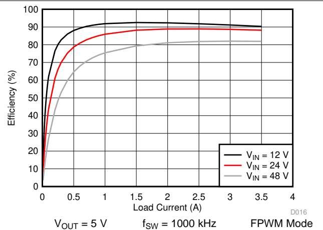
图 28. LM76003-Q1 Efficiency
