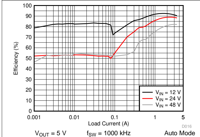
图 27. LM76003-Q1 Efficiency
