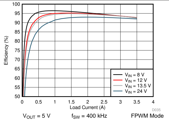
图 26. LM76003-Q1 Efficiency
