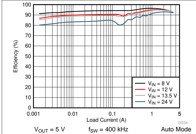
图 25. LM76003-Q1 Efficiency
