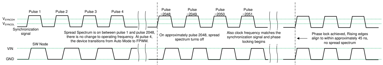
图 8-12. 同步过程
