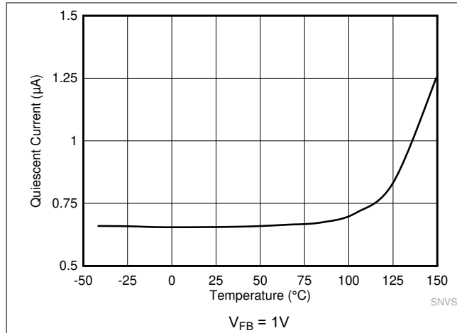
图 7-1. 非开关输入电源电流
