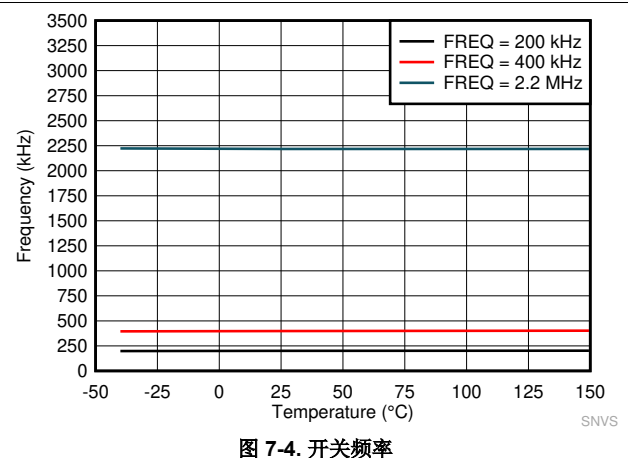
图 7-4. 开关频率
