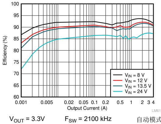
图 9-5. LMQ62440-Q1 效率
