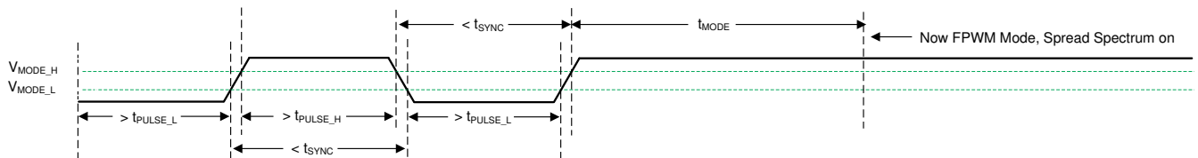
图 8-11. 从 SYNC 模式转换到 FPWM 模式
