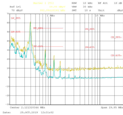
F_{SW} = 400\text{ kHz} V_{OUT} = 5V I_{OUT} = 5A 测试频率：150 kHz 至 30 MHz
