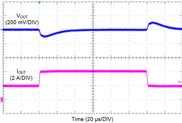
V_{OUT} = 5V F_{SW} = 2100\text{ kHz} 自动模式 I_{OUT} = 2A 至 4A 至 2A V_{IN} = 13.5V T_R = T_F = 2\mu s
