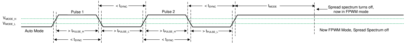
图 8-9. 从自动模式转换到 FPWM 模式时禁用展频
