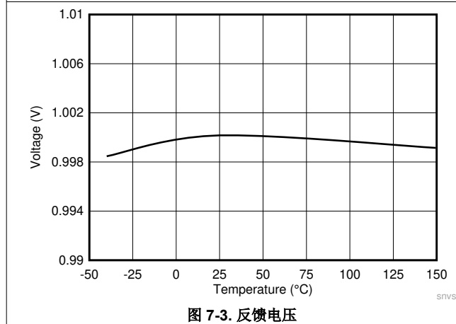
图 7-3. 反馈电压
