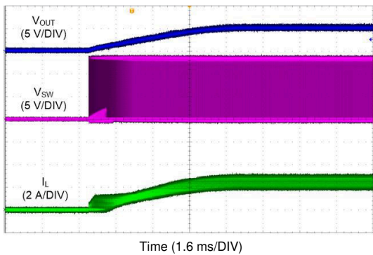
图 9-19. LMQ62440-Q1 在 3.25A 时启动
