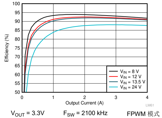
图 9-6. LMQ62440-Q1 效率
