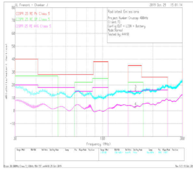
V_{OUT} = 5V F_{SW} = 400\text{ kHz} I_{OUT} = 5\text{ A} 测试频率：30 MHz 至 300 MHz
