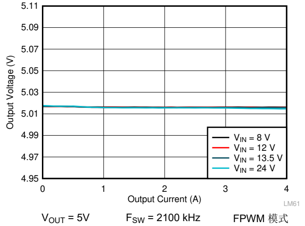
图 9-12. LMQ62440-Q1 负载和线性调整率
