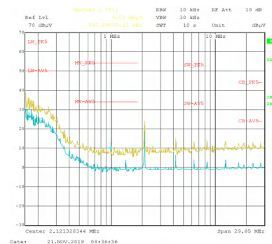
F_{SW} = 2100\text{ kHz} V_{OUT} = 5V I_{OUT} = 5\text{ A} 测试频率：150 kHz 至 30 MHz
