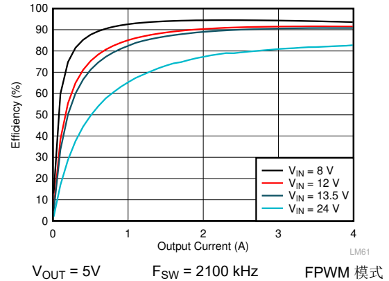
图 9-8. LMQ62440-Q1 效率
