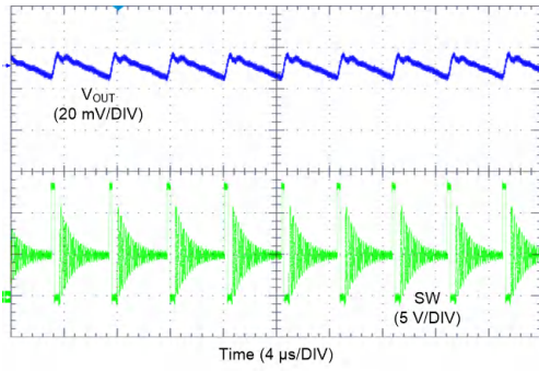
图 9-17. LMQ62440-Q1 开关波形和 V_{OUT} 纹波
