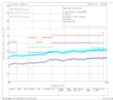
V_{OUT} = 5V F_{SW} = 400\text{ kHz} I_{OUT} = 5\text{ A} 测试频率：300 MHz 至 1 GHz
