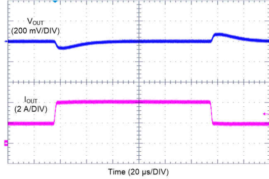
V_{OUT} = 3.3V F_{SW} = 2100\text{ kHz} 自动模式 I_{OUT} = 2A 至 4A 至 2A V_{IN} = 13.5V T_R = T_F = 2\mu s
