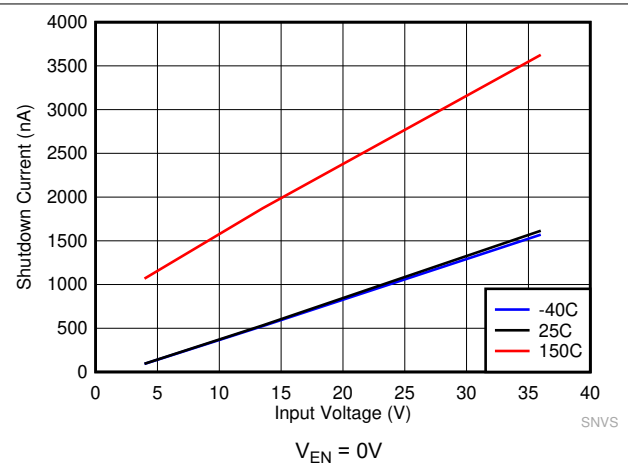
图 7-2. 关断电源电流
