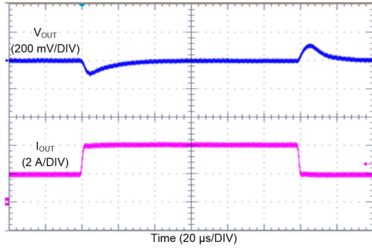
V_{OUT} = 3.3V F_{SW} = 400\text{ kHz} 自动模式 I_{OUT} = 2A 至 4A 至 2A V_{IN} = 13.5V T_R = T_F = 2\mu s
